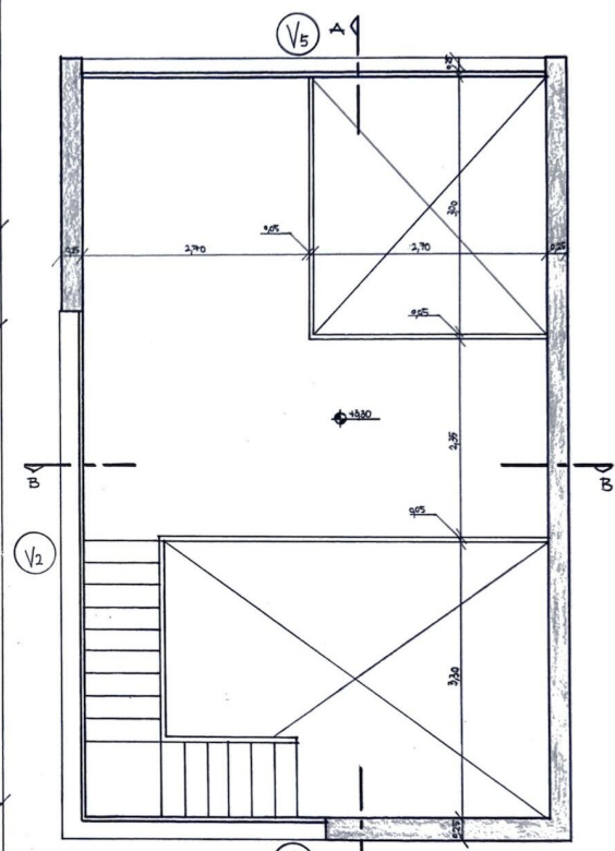
PLANTA ALTA ESC 1:50
