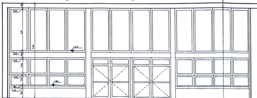
CORTE A-A ESK 1:50
