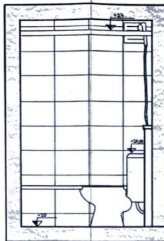
CORTE B-B Esc. 1:20
