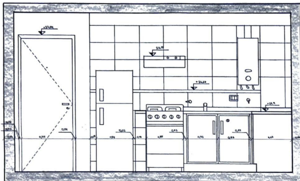
CORTE A-A Esc. 1:50
