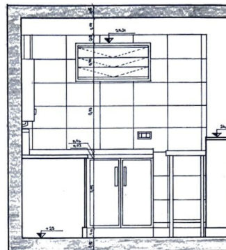
CORTE B-B Esc. 1:50
