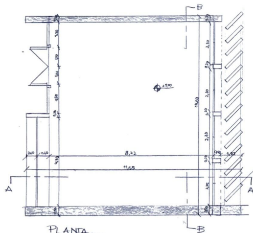
PLANTA ESC. 1:100
