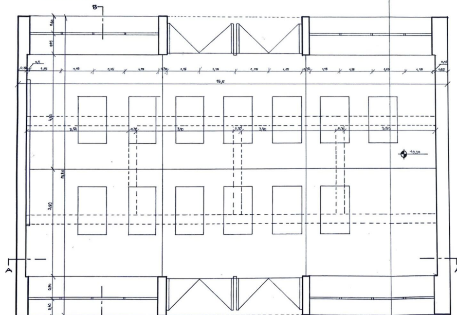
PLANTA ESK 1:50
