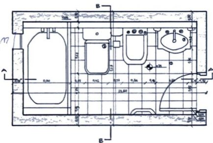
PLANTA Esc. 1:20
