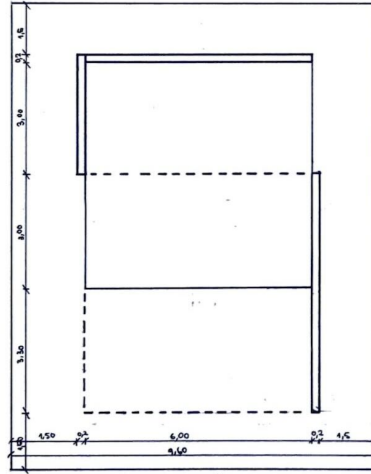
PLANTA Esc 1:100
