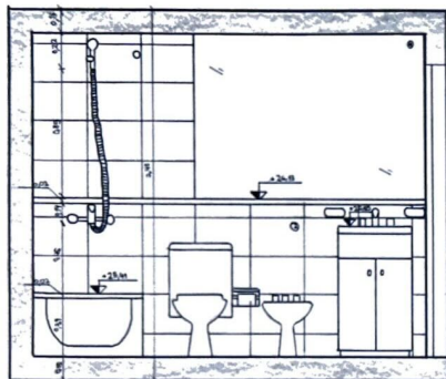
CORTE A-A Esc. 1:20
