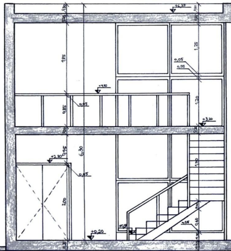
CORTE B-B ESC 150
