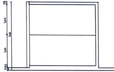
CORTE B-B Esc 1:100
