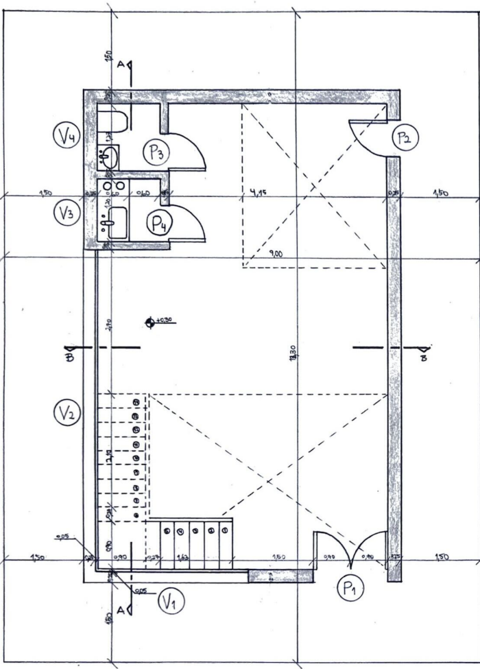
PLANTA BAJA ESC 1:50
