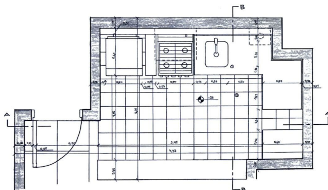
PLANTA Esc. 1:50
